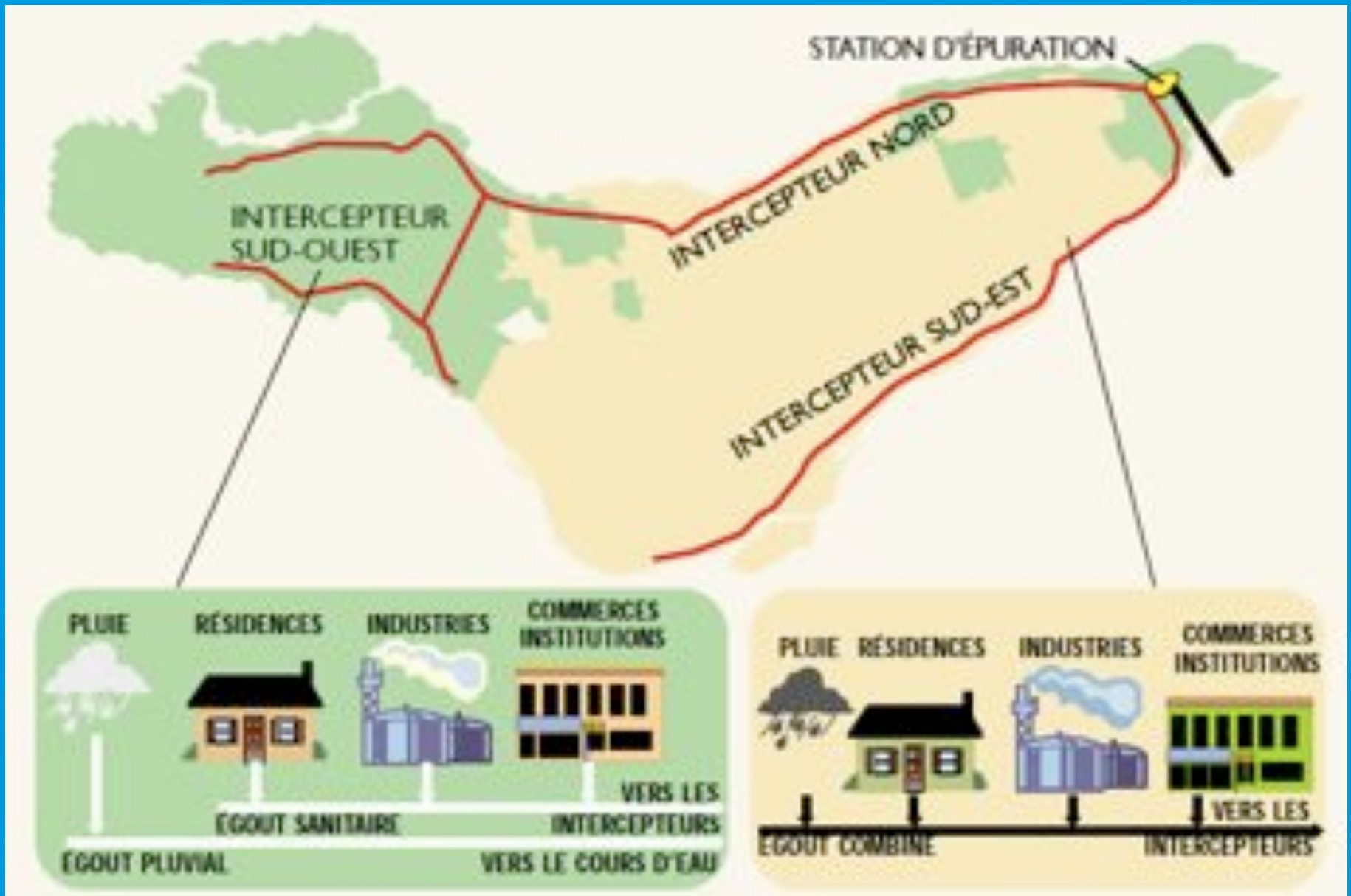
Station d'épuration Jean-R. Marcotte, Montréal
